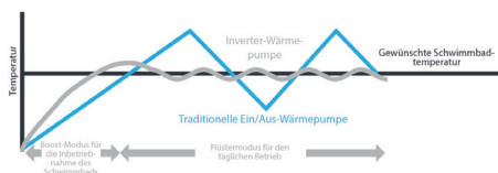
Diagramm der Temperaturregelung
